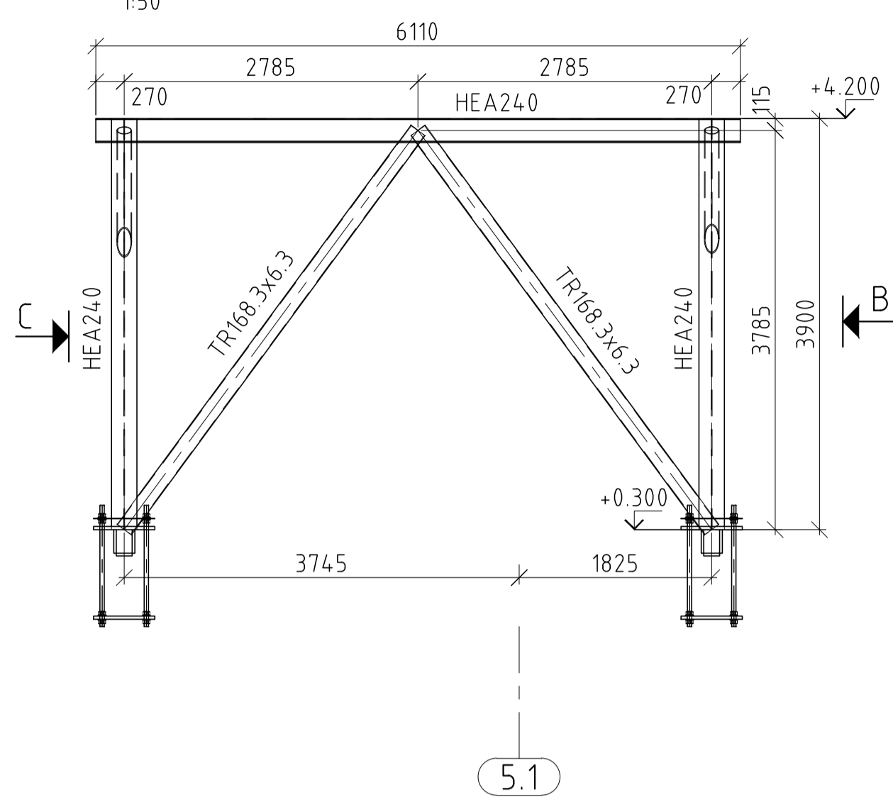
PODPORA 9 POHLED A 150
