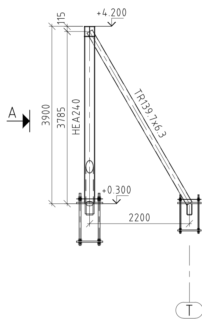
PODPORA 9 POHLED B 150
