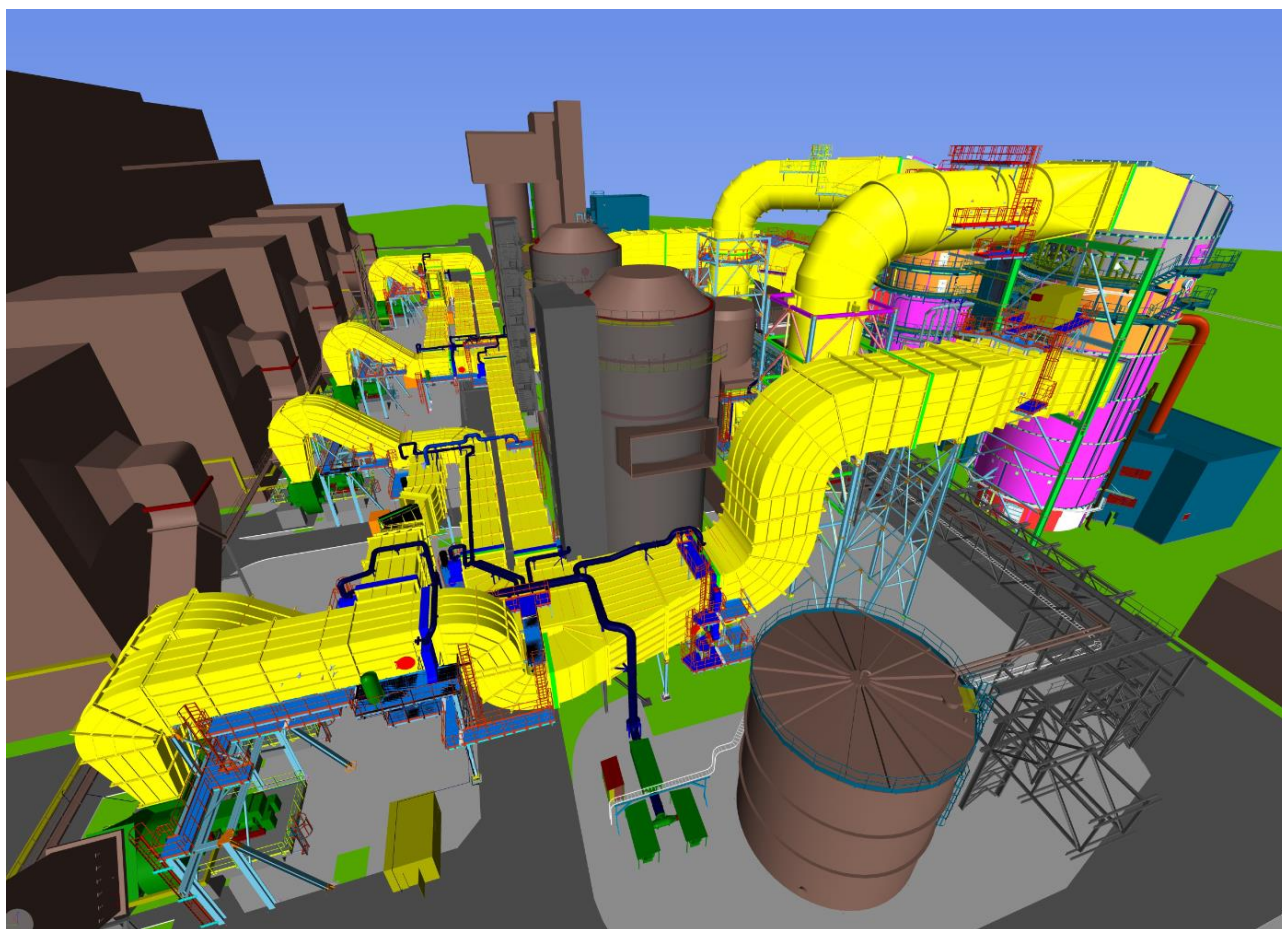
Obr. 2 Celková dispozice s označením řešené oblasti
